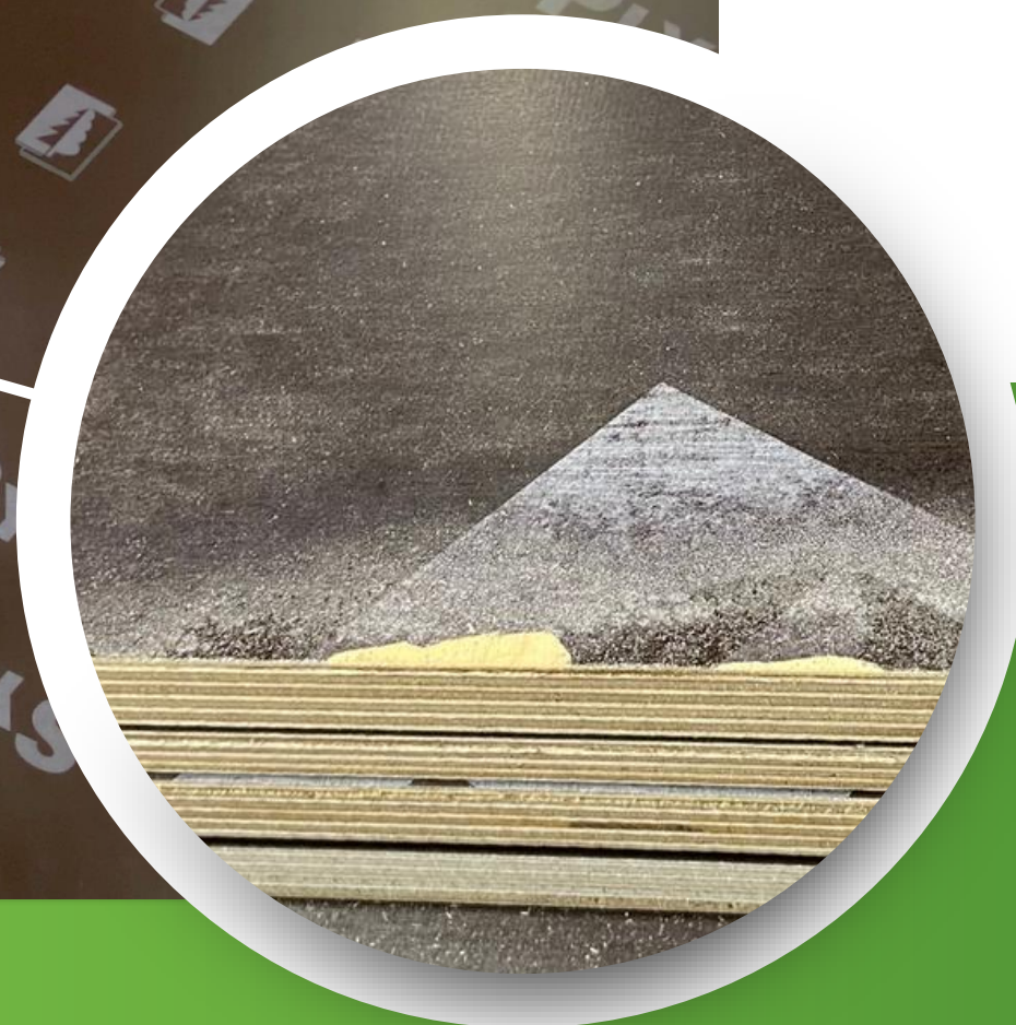
Осыпание пленки
