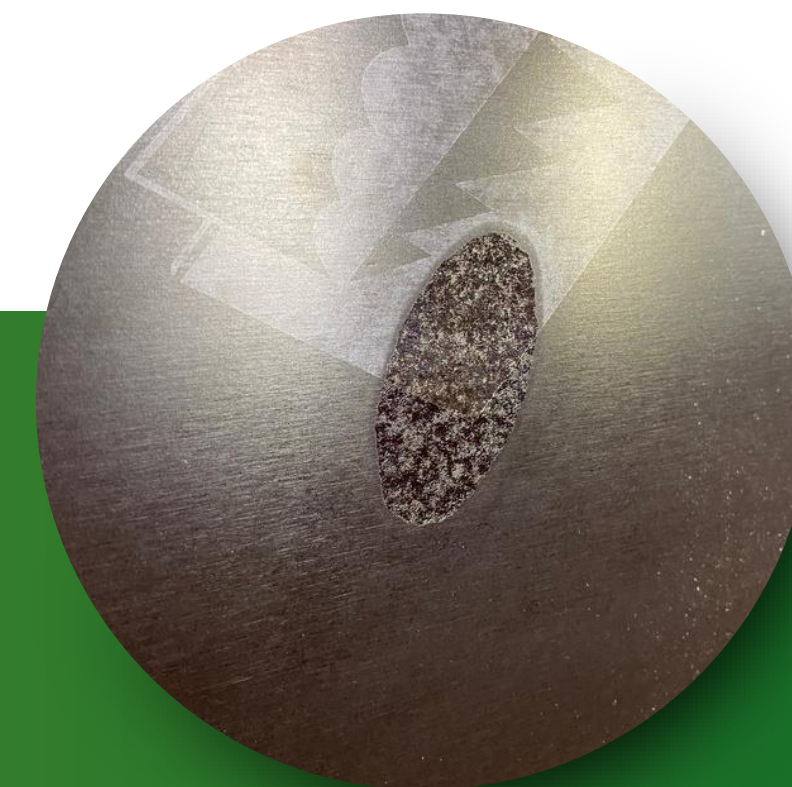
Прогар по доработанному дефекту (вставка)
