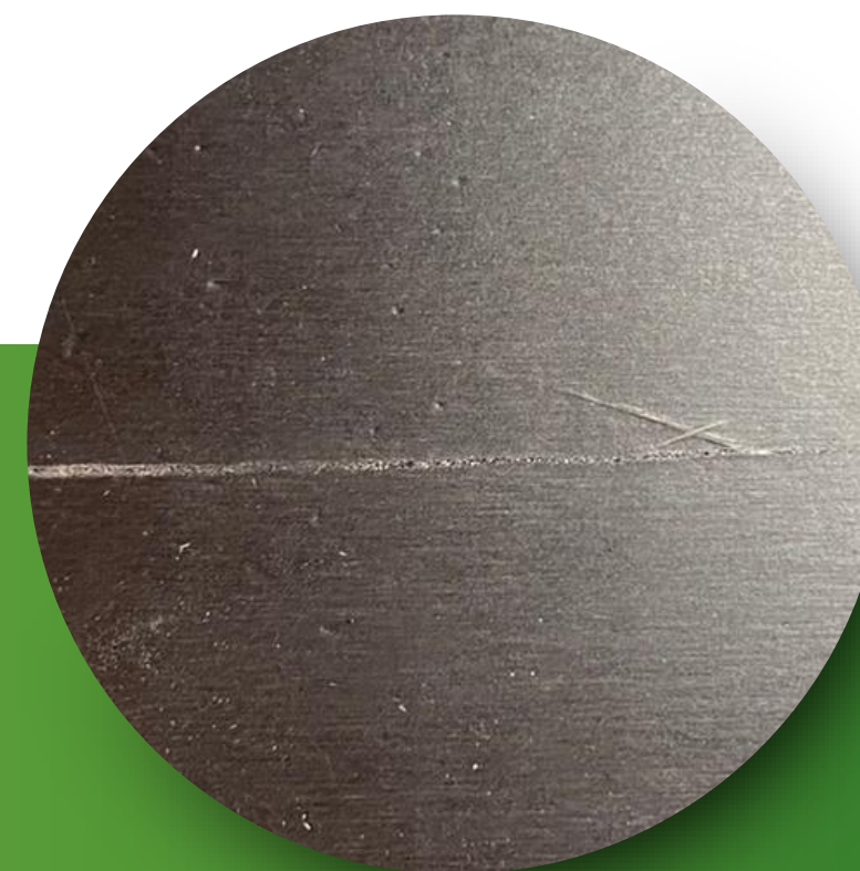
Прогар по недоработанному дефекту (трещина)
