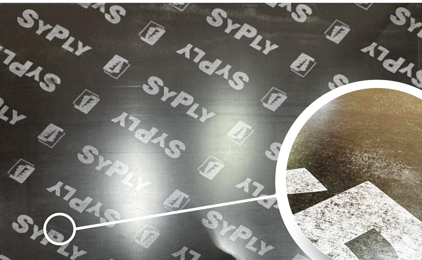
Прогар по внутреннему дефекту
